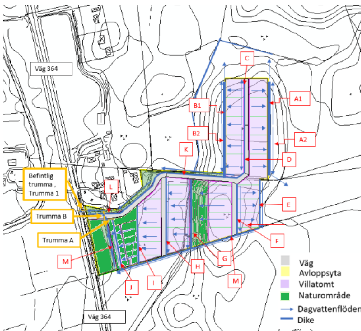
Figur 23. Ugefärlig skiss över dagvattenflöden och rinnvägar
