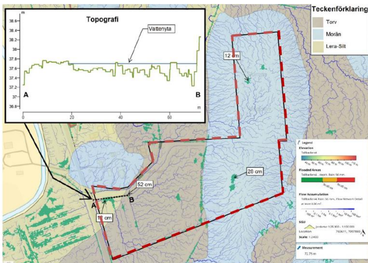
Figur 31. Instängda områden med risk för översvämning i befintlig situation baserat på 100-årsregn (56 mm). Planområdet markeras med röd streckad linje. Källa, VA- och dagvattenutredning, WSP.
