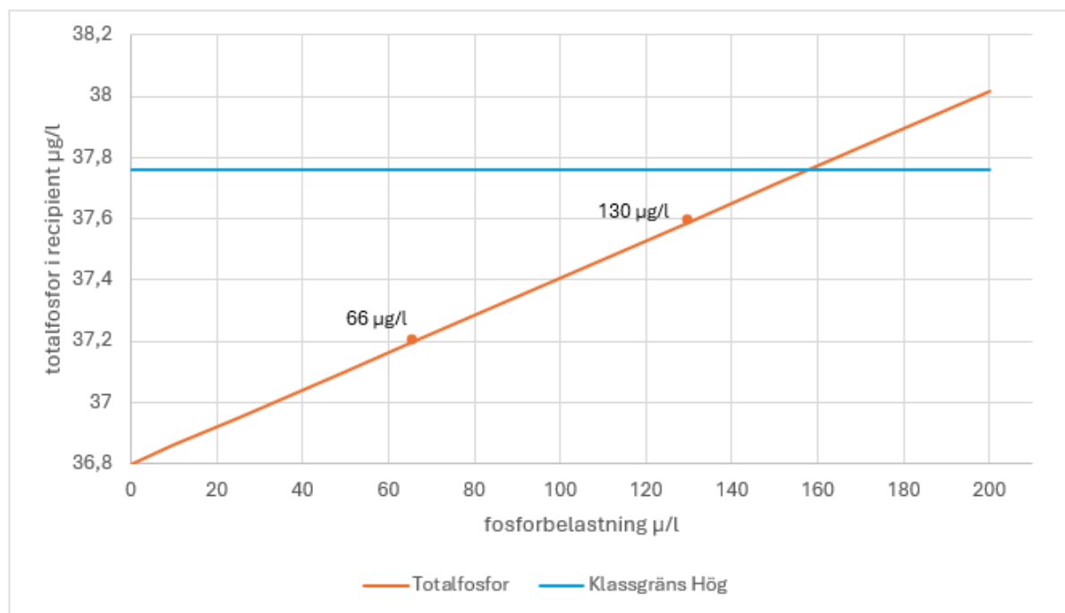
Figur 14. Den totala halten fosfor i recipienten (µg/l) vid olika utsläpp av fosforhalter (µg/l). Blå linje anger klassgränsen för Hög status i recipienten vilket inte får överstigas för att inte försämra statusen.
