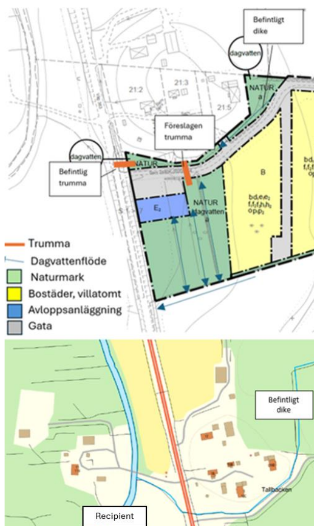
Figur 22. Trummor och befintliga diken (Befintligt dike är blå heldragen linje som kopplar an till Fällforsån via trumma under länsväg 364).
