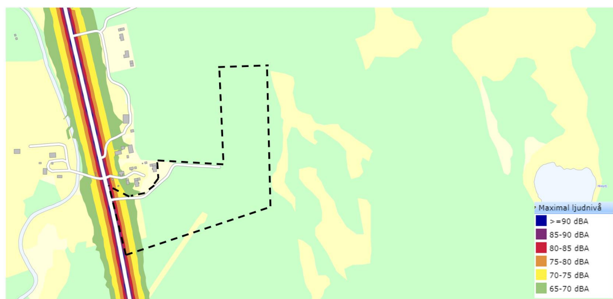
Figur 29. Maximal ljudnivå, dBA vägbuller. Planområdet är markerat med svart streckad linje
