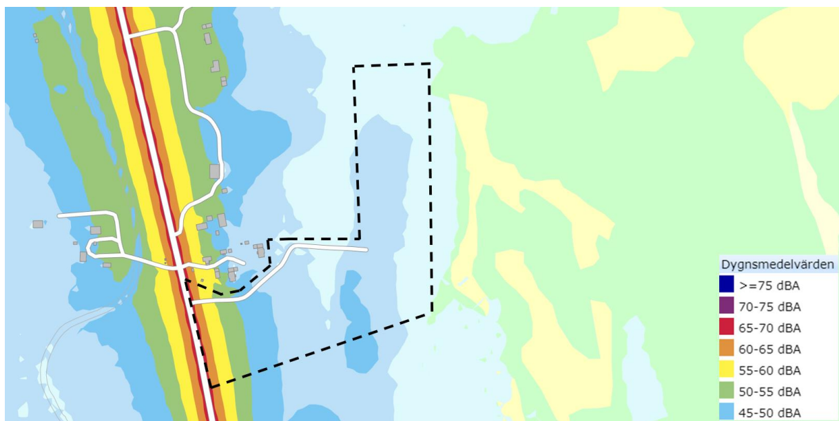
Figur 28. Dygnsmedelvärden, dBA, vägbuller. Planområdet är markerat med svart streckad linje
