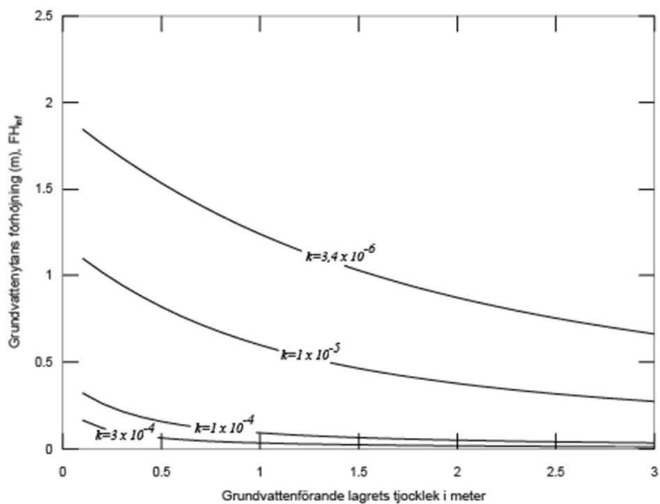
Figur 4. Grundvattennivåns förhöjning ( FH_{inf} ) som funktion av grundvattenförande lagrets tjocklek vid några olika k -värden. Kurvorna är beräknade baserat på metod beskriven av Finnemore 1993 2 .
