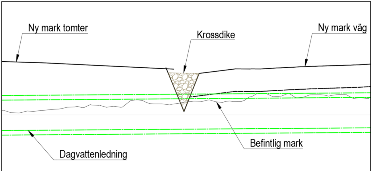
Figur 10. Utformningsförslag 1: kritisk punkt för kulvertering av bäck projekterad mot tillgänglig laserdata som höjdreferens.
